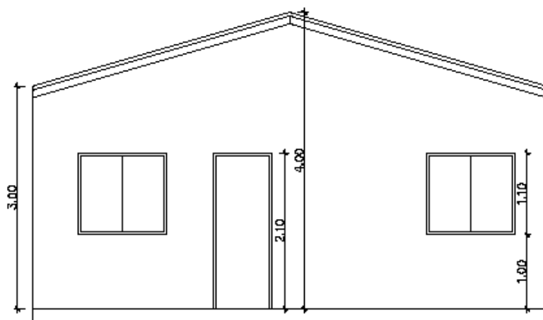
FACHADA FRONTAL
