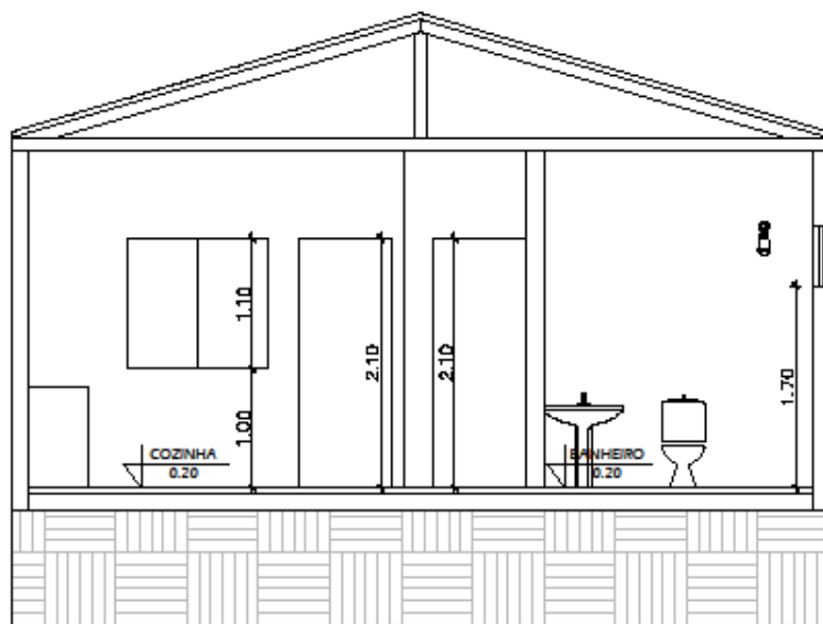
PLANTA DE CORTE AA
